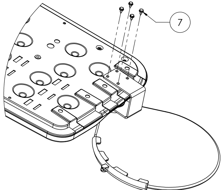
50153 x1 (Steel)
